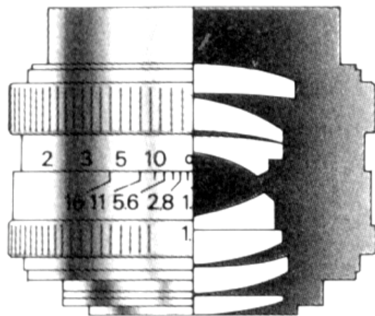
“Κανονικός” φακός 50mm
