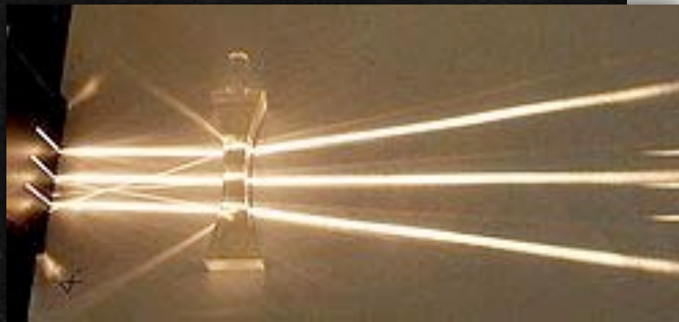
Αμφίκοιλος ή αποκεντρωτικός φακός
